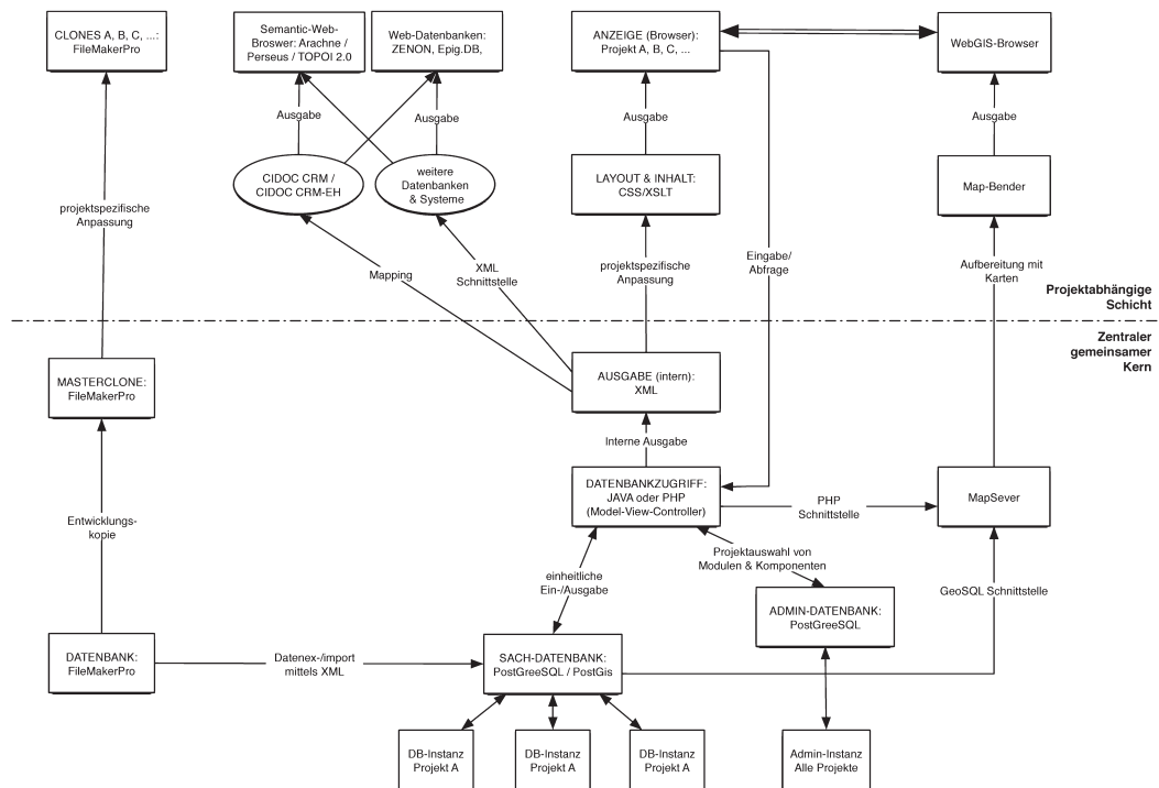
Abb. 6: Softwarearchitektur der geplanten Webapplikation.
