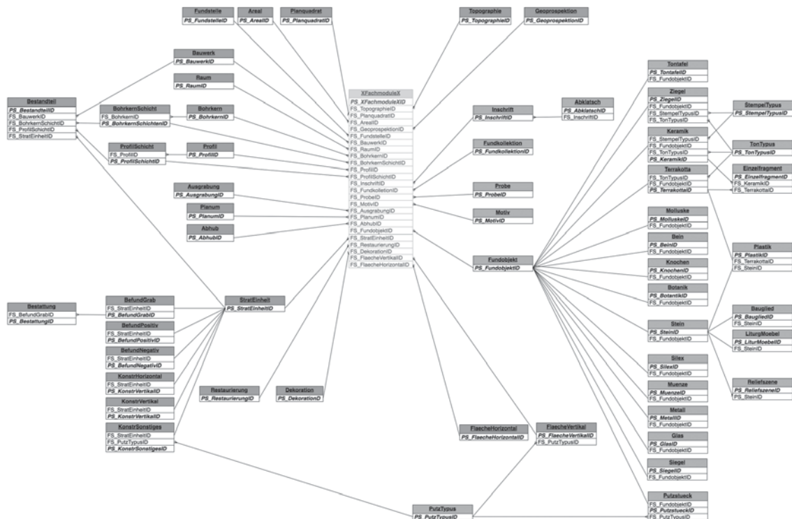
Abb. 4: Vereinfachtes Datenmodell mit zentraler Kreuztabelle.
